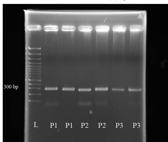
شکل ۱: الکتروفورز محصولات PCR از آزمون دوم ژن کانکسین ۲۶ بر روی ژل آگارز. L مارکر ۱۰۰ جفت باز می‌باشد. P1، P2 و P3 به ترتیب نشان‌دهنده محصولات PCR جفت پرایمر اول (F,3R۱)، جفت پرایمر دوم (F,15R۱۰) و جفت پرایمر سوم (F,5R۱) می‌باشد.
